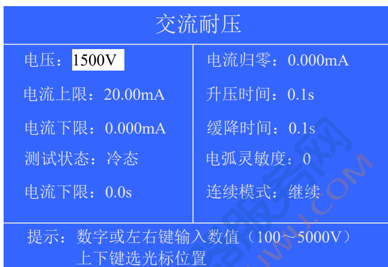
图 5.7 交流耐压测试设置
